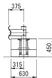
[標準タイプ]
