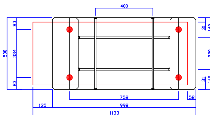
E500 (連結ボルト668mmにカット)
