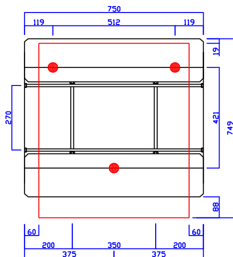
E750 (連結ボルト331mmにカット)
