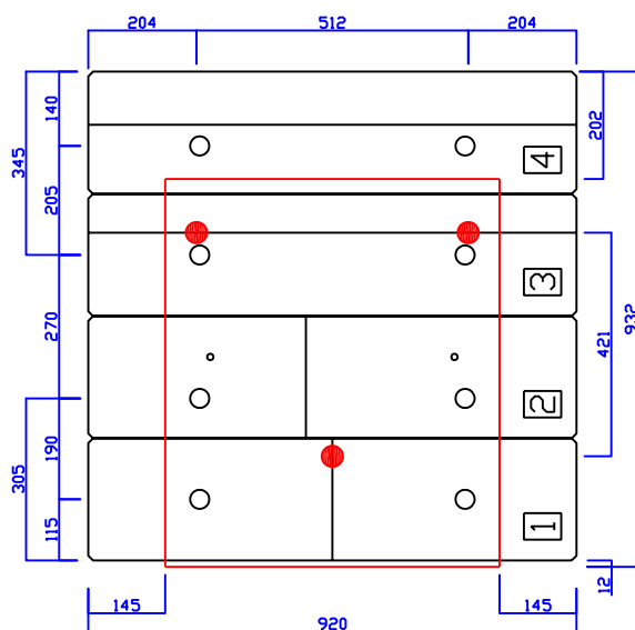
HE920 Type A (タンクを壁から離したい場合)
