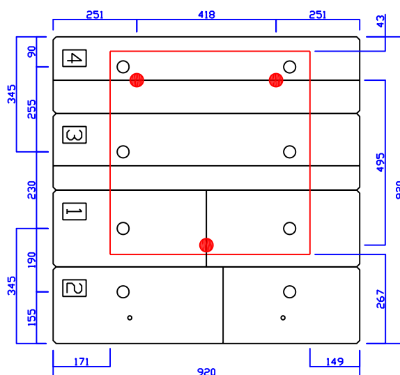
HE920 Type B (タンクを壁に近づけたい場合)
