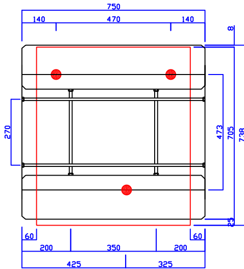
E750 (連結ボルト383mmにカット)
