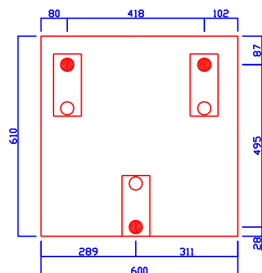
メンテナンス面 タンク形状・アンカーピッチ
