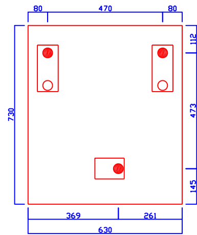
メンテナンス面 タンク形状・アンカーピッチ
