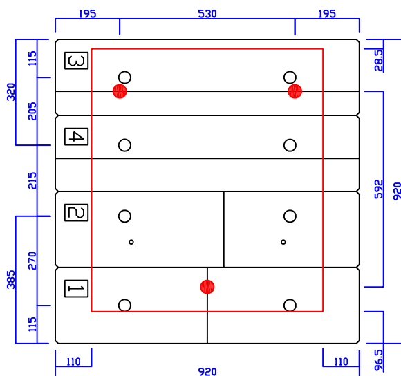
HE920 Type A (タンクを壁から離したい場合)
