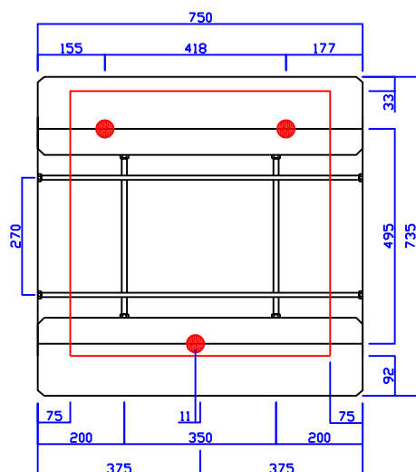
E750 (連結ボルト405mmにカット)
