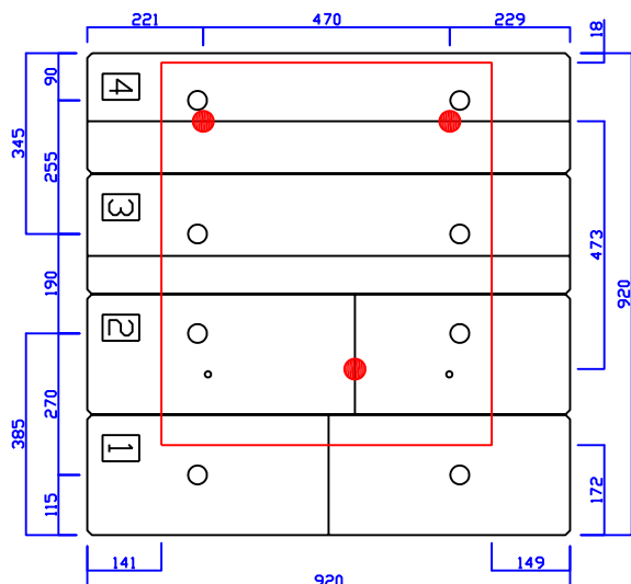
HE920 Type B (タンクを壁に近づけたい場合)
