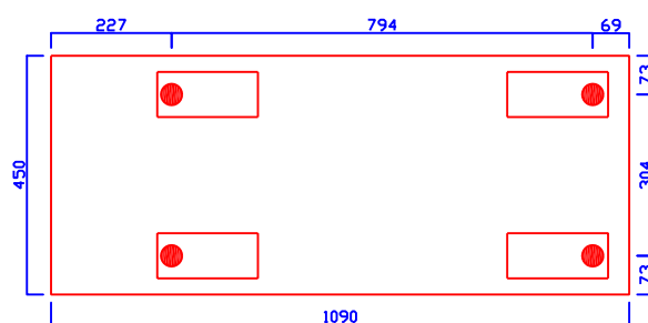
タンク形状・アンカーピッチ
