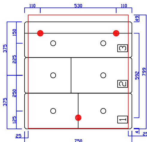
メンテナンス面 タンク形状・アンカーピッチ
