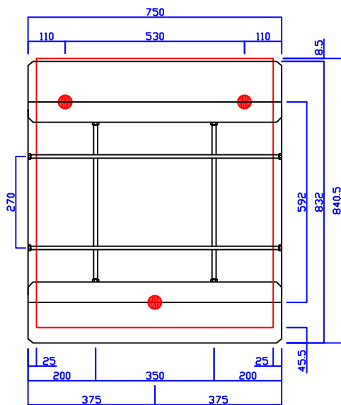
E750 (連結ボルト502mmにカット)
