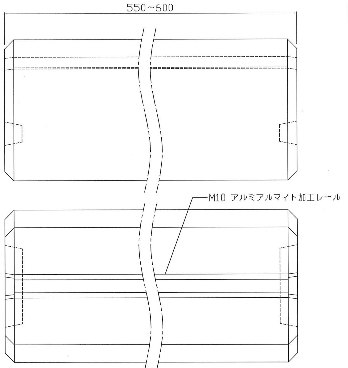
タイガーベース L550~600 製品図
